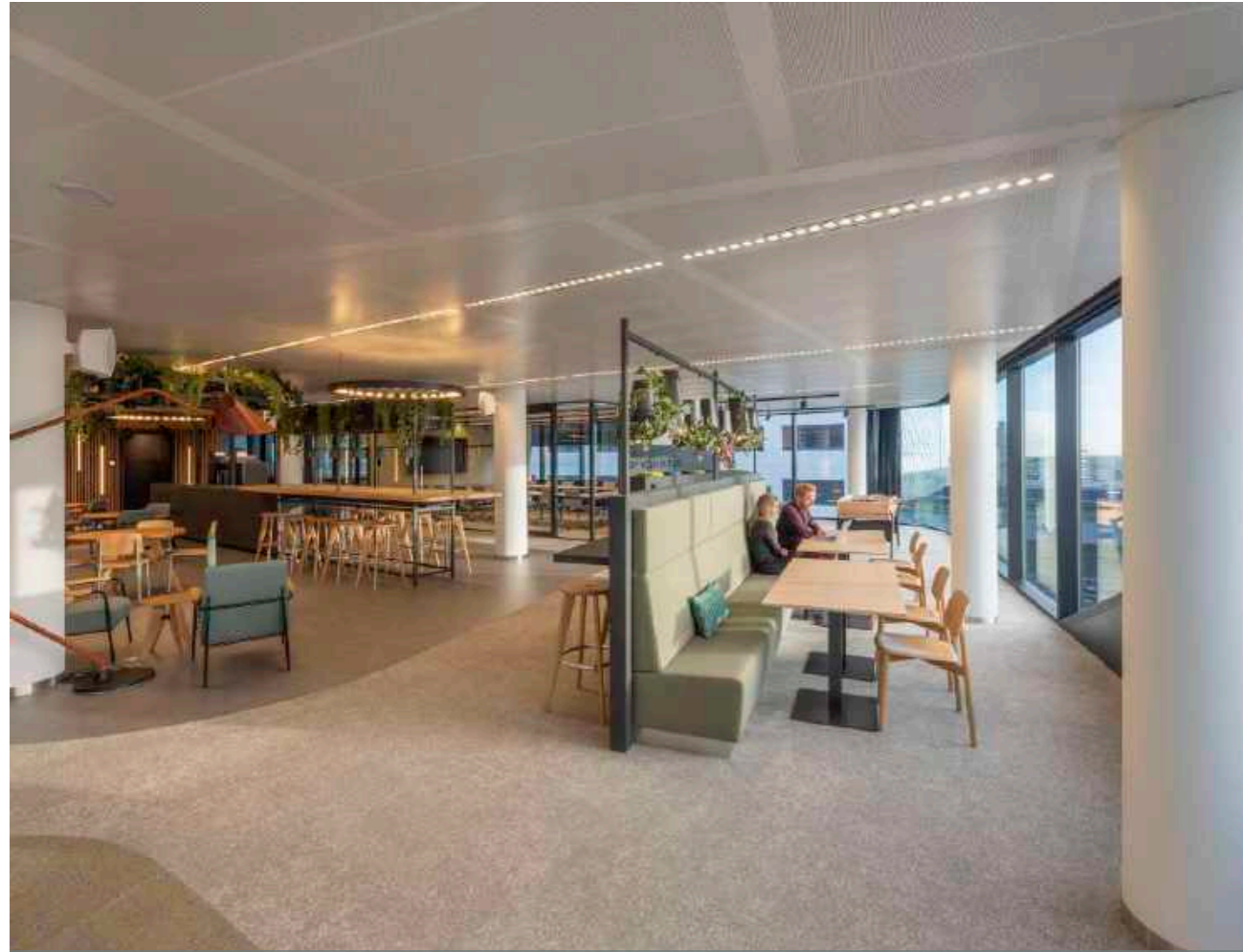
WTC - UTRECHT
